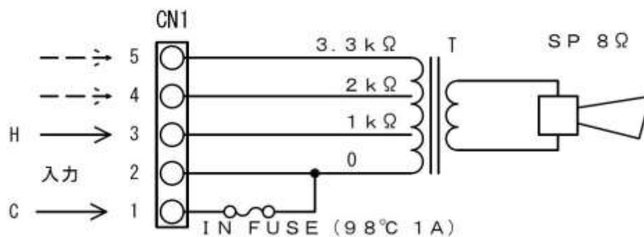
内部接続図
