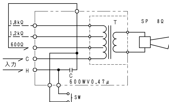
内部接続図
