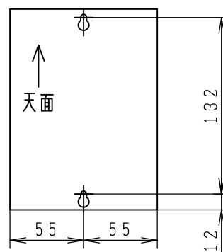
取付け穴図 (底面) 尺度 1/4
