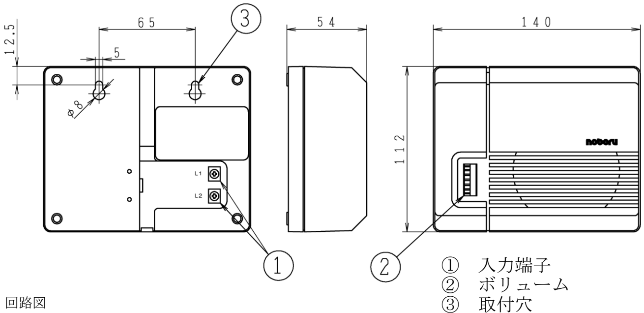
外観図
