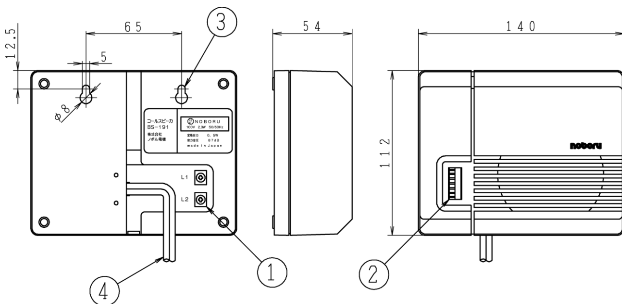
外観図
