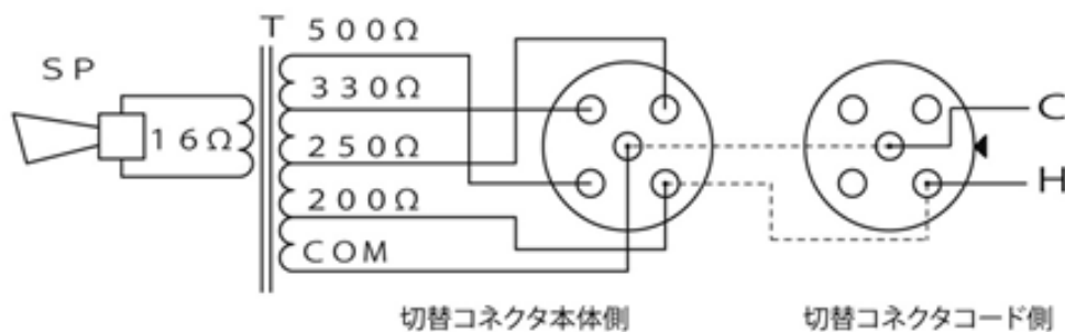
出荷時の結線図
