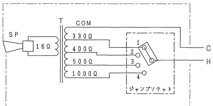
回路図
