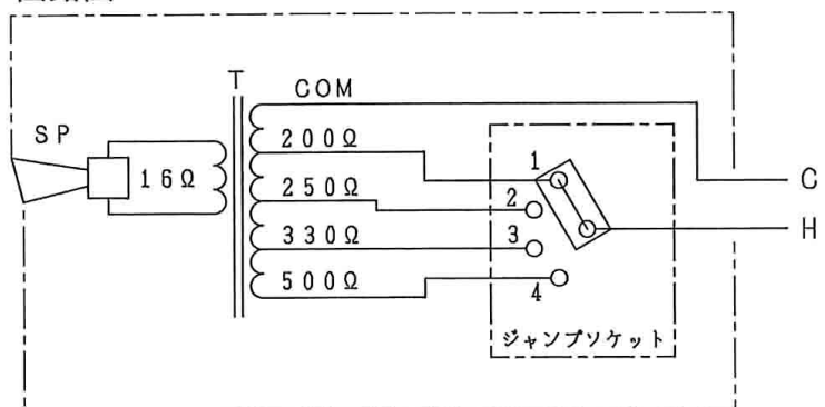
回路図
