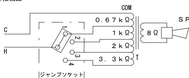
内部接続図
