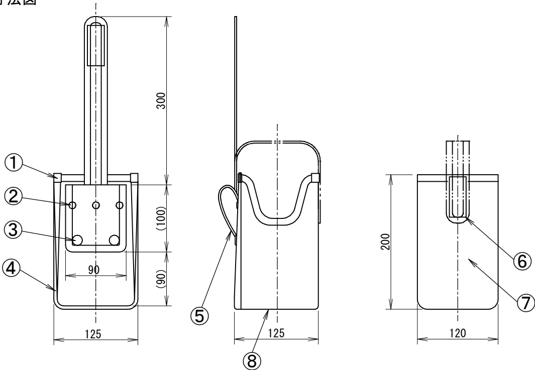
○外観寸法図
