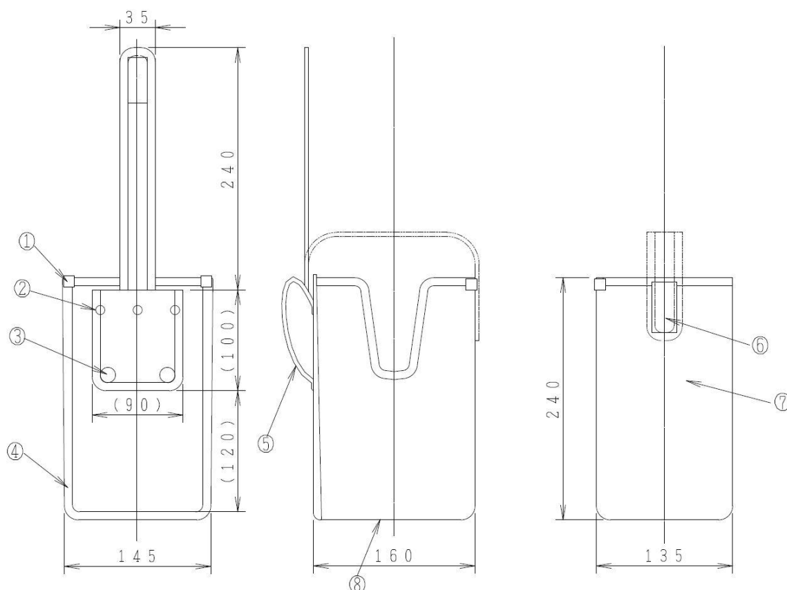
○外觀寸法図
