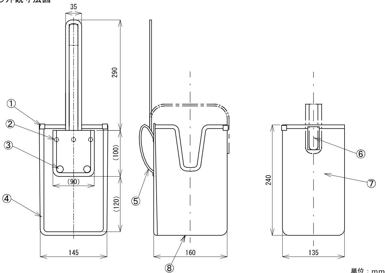
○外観寸法図
