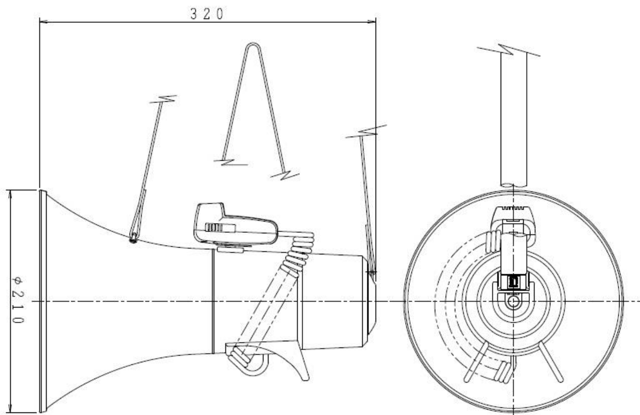
外観図
