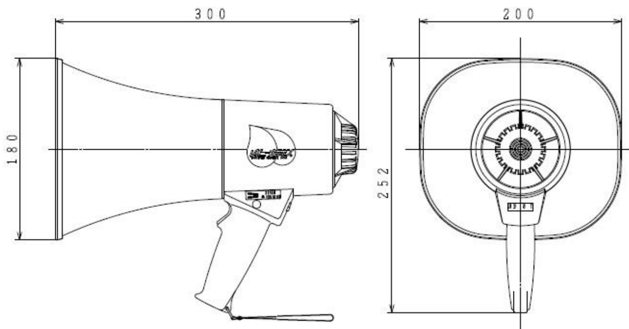
外観図
